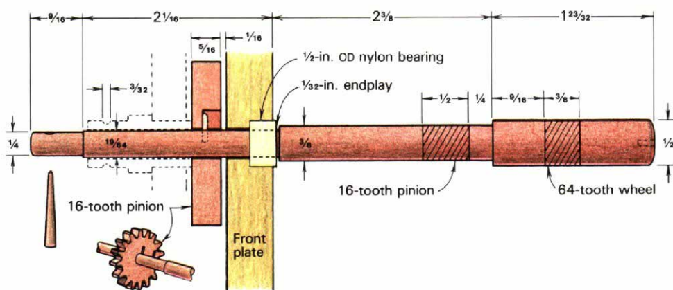
Center arbor
